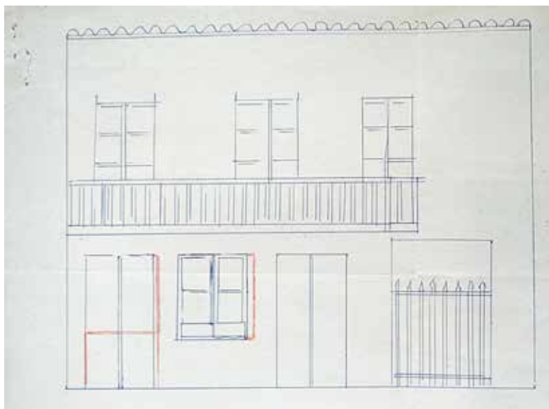
64 Alçat façana principal. Llicència d'obres, 1962. Arxiu Municipal Torroella de Montgrí.
