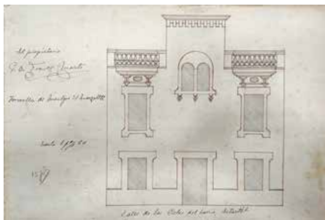
90 Alçat de la façana principal, 1922. 32 x 22 cm. Arxiu Municipal de Torroella de Montgrí.
