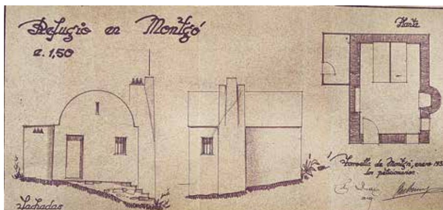
29 Alçat de façanes i planta. 1935. Arxiu Municipal de Torroella de Montgrí.
