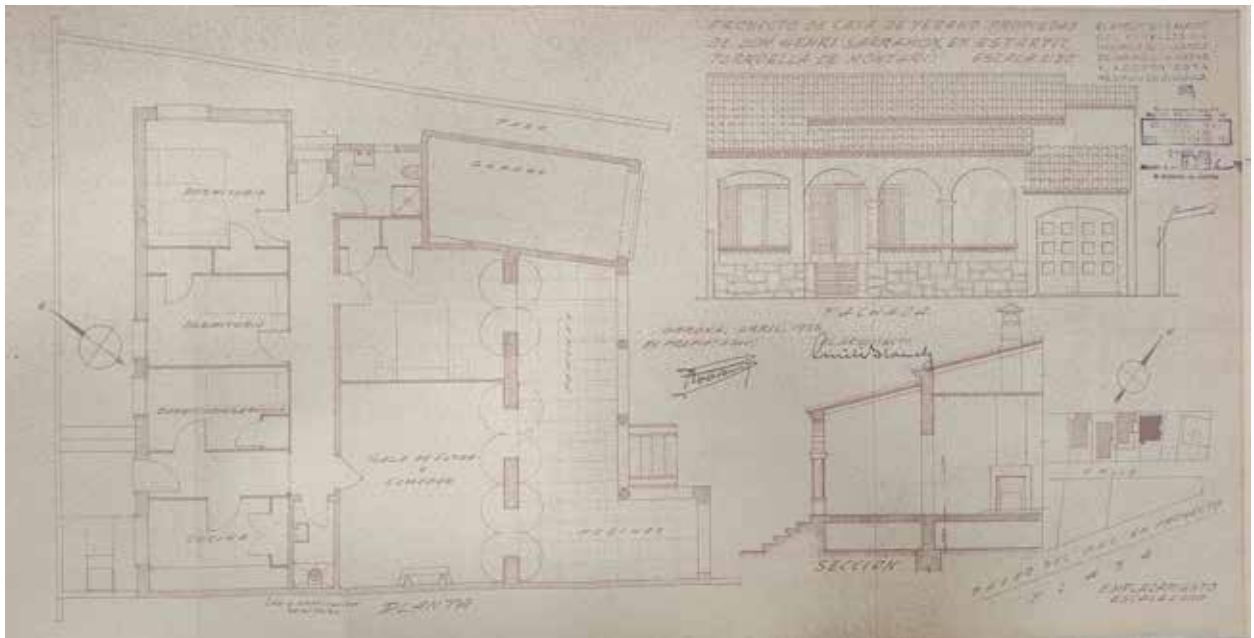
131 Alçats façana, secció i planta de la casa projectada per Emili Blanch per a Henri Sarramon. 1956. Arxiu Municipal de Torroella de Montgrí.
