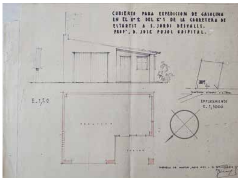
135 Alçat i secció del cobert de la benzinera de l'Estartit. Arxiu Municipal de Torroella de Montgrí.
