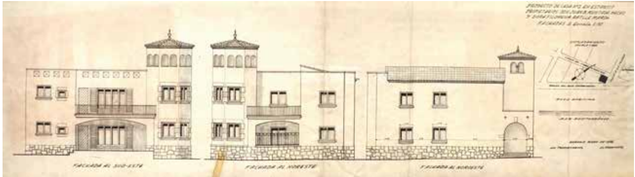
130 Alçats façanes sud-est i nord-est de la casa projectada per Emili Blanch per a Joan Baptista Muntada i Filomena Batlle. 1956. Arxiu Municipal de Girona.
