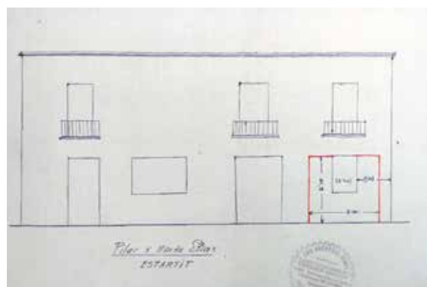
46 Alçat façana principal. Llicència d'obres, 1960. 28 x 21 cm. Arxiu Municipal Torroella de Montgrí.
