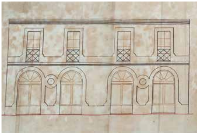
52 Alçat façana principal. Llicència d'obres, 1876. Arxiu Municipal Torroella de Montgrí.
