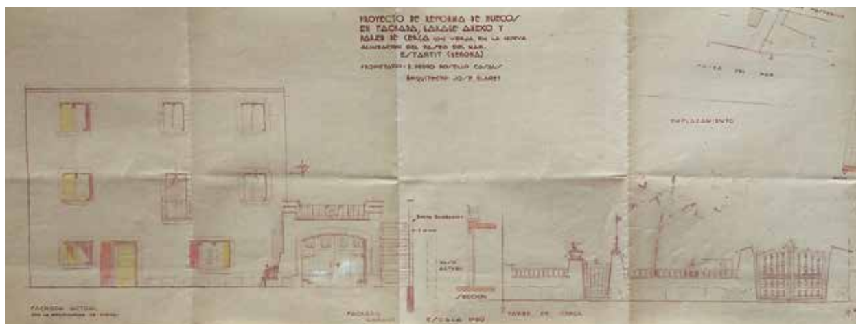
96 Alçat de la façana principal i tanca del jardí, 1954. 99 x 29 cm. Arxiu Municipal de Torroella de Montgrí.
