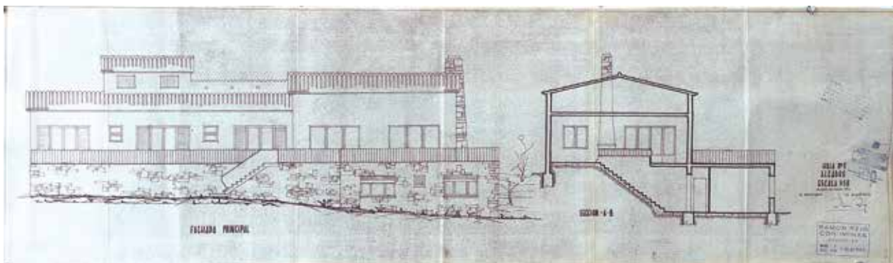
124 Alçat i secció de la façana principal de la casa projectada per a Santiago Fisas. 106 x 31 cm. Arxiu Municipal de Torroella de Montgrí.
