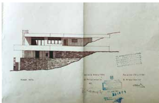
139 Alçat nord pel projecte de la casa de Werner Straub. 1964. 62 x 38 cm. Arxiu Municipal de Torroella de Montgrí.
