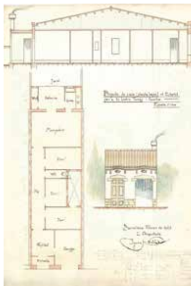
77 Secció longitudinal i planta del projecte de la casa d'Isidre Torres. 1923. Arxiu Comarcal de l'Anoia.
