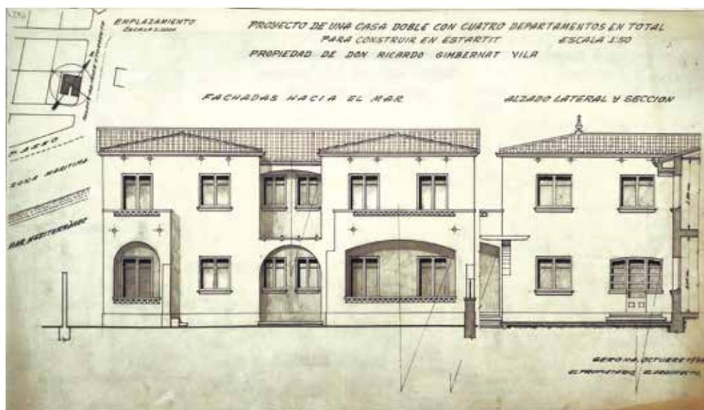
129 Alçats façanes principal, lateral i secció de la casa plurifamiliar projectat per Emili Blanc per a Ricard Gimbernàt i Dolors Pujol. 1955. Arxiu Municipal de Girona.
