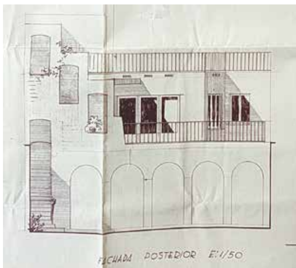
56 Alçat façana posterior. Llicència d'obres, 1960. Arxiu Municipal Torroella de Montgrí.
