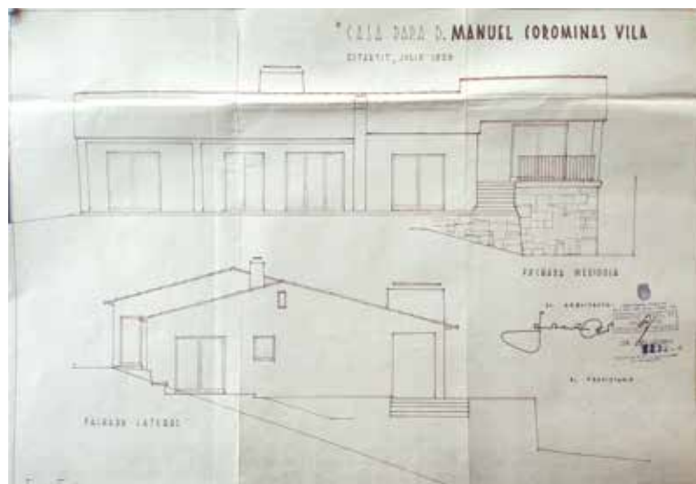
122 Alçat de la façana sud i lateral de la casa projectada per a Manel Corominas Vila. 52 x 36,5 cm. Arxiu Municipal de Torroella de Montgrí.
