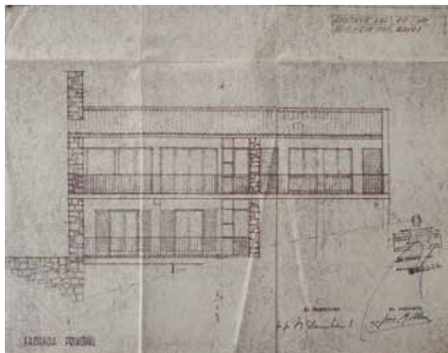
136 Alçat de la façana principal pel projecte de la casa de Vladimir Raitz. 1961. 52 x 43 cm. Arxiu Municipal de Torroella de Montgrí.
