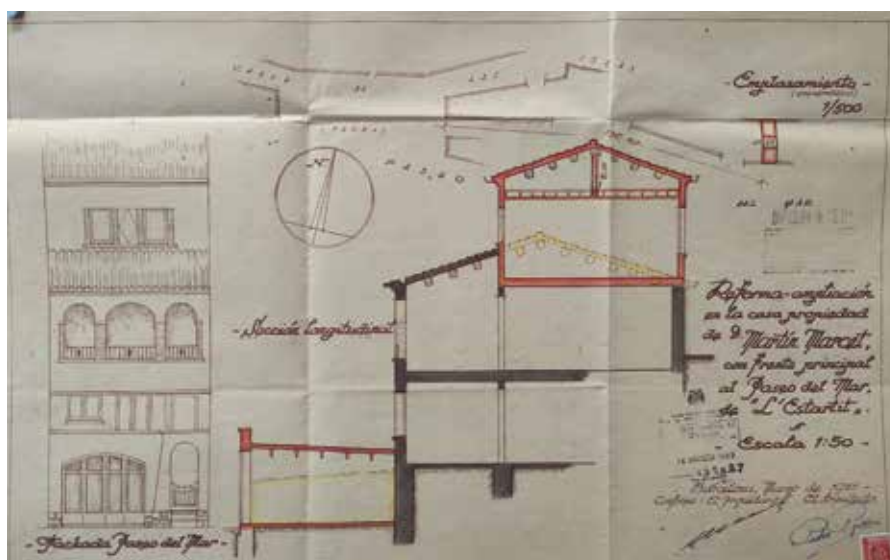
97 Façana principal i secció. 1955. 55 x 35 cm. Projecte casa Martí Marcet. Arxiu Municipal de Torroella de Montgrí.
