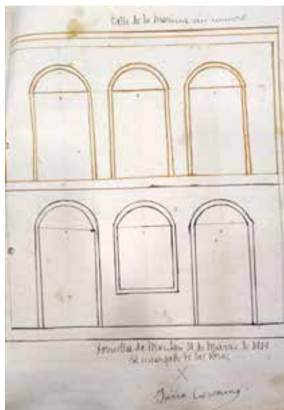
63 Alçat façana principal. Llicència d'obres, 1919. Arxiu Municipal Torroella de Montgrí.
