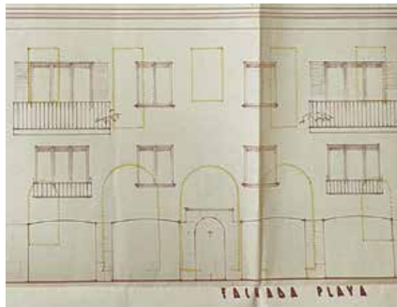
53 Alçat façana principal. Llicència d'obres, 1960. Arxiu Municipal Torroella de Montgrí.
