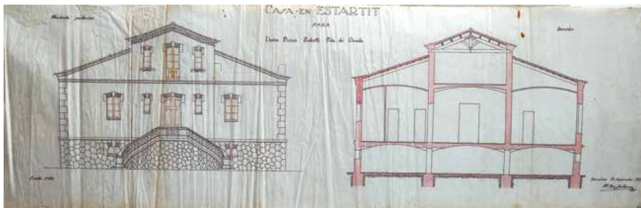
58 Alçat de la façana posterior del projecte Casa Boada de l'arquitecte Josep Maria Miró. 1917. Col·lecció família Trill.
