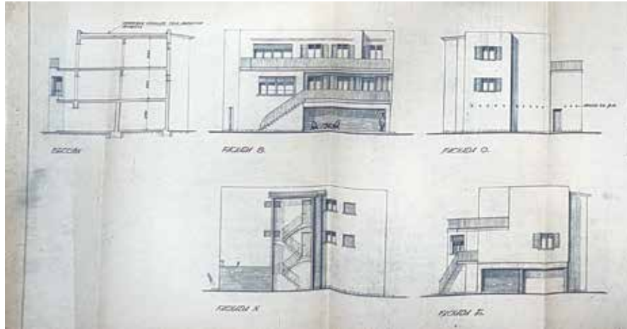
113 Façanes i secció. 1961. Projecte reforma de la casa de Pilar Florensa. Arxiu Municipal de Torroella de Montgrí.
