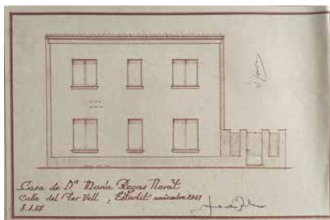
104 Alçat de la façana principal de la casa de Walda Pla. 1951. Arxiu Municipal de Torroella de Montgrí.
